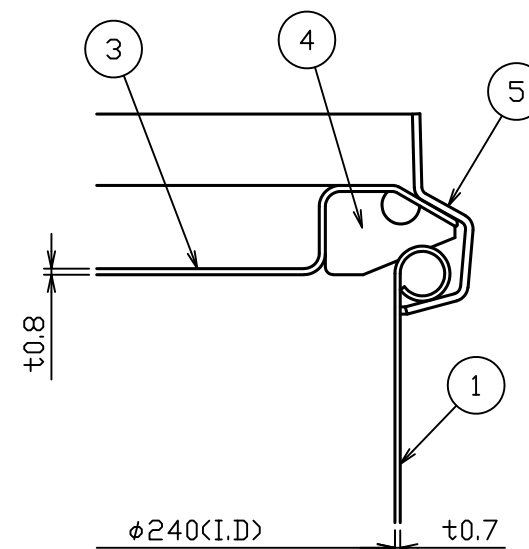
A部詳細図 S = 1 : 1
