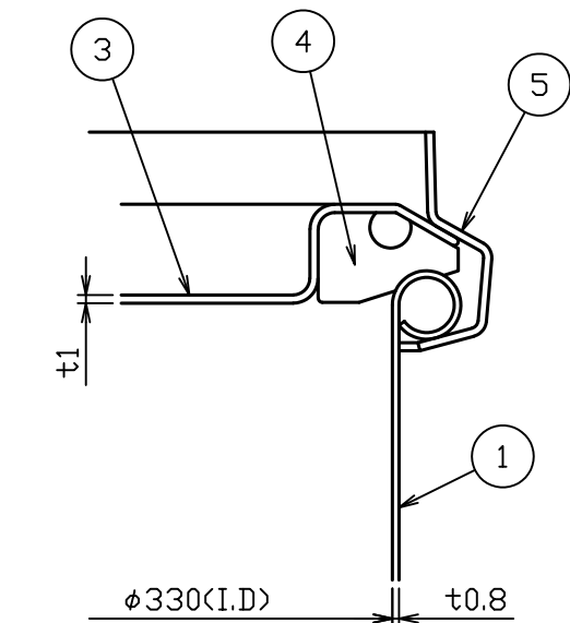
A部詳細図 S = 1 : 1
