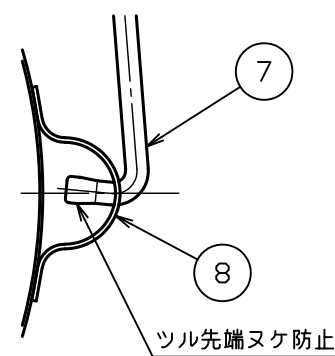
△B部詳細図 S = 1 : 2
