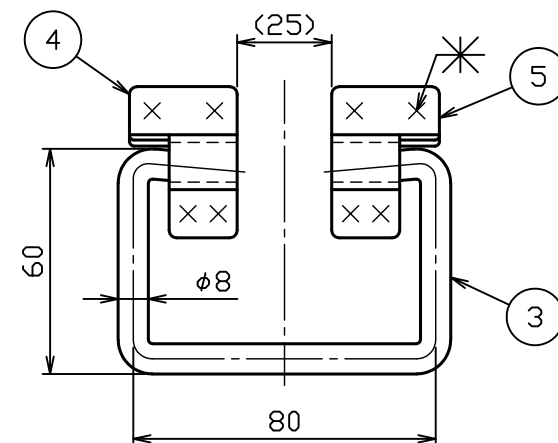
把手部詳細図 S = 1 : 2
