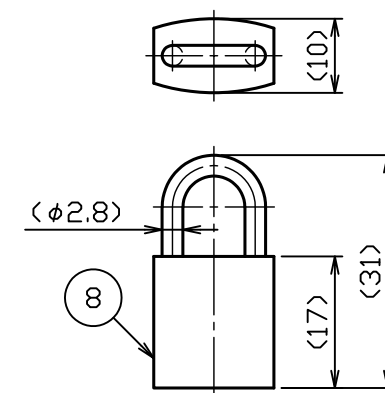
南京錠 S = 1 : 1
