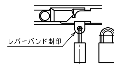
C部詳細図 S = 1 : 2
