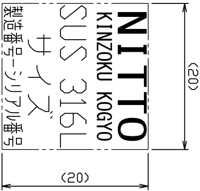
レーザーマーク詳細図
