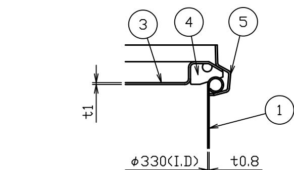
A部詳細図 S = 1 : 2
