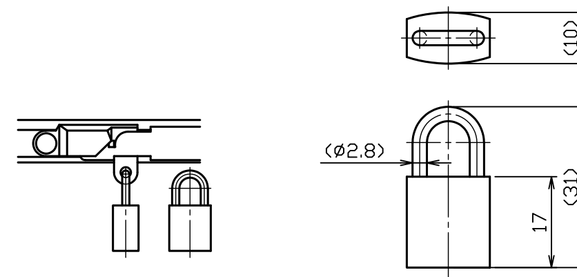
C部詳細図 S = 1 : 2 南京錠 S = 1 : 1
