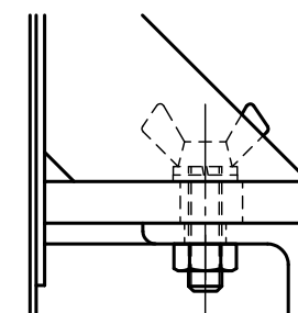
蝶ボルト部詳細図 S = 1 : 2
