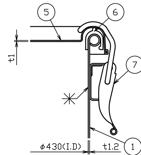
A部詳細図 S = 1 : 2
