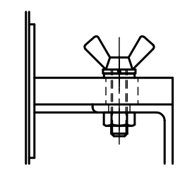
△蝶ボルト部詳細図 S = 1 : 2
