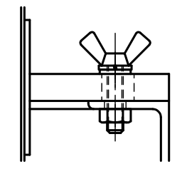
△蝶ボルト部詳細図 S = 1 : 2
