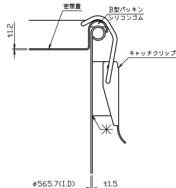
A部詳細図 S = 1 : 2
