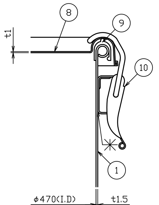
A部詳細図 S = 1 : 2
