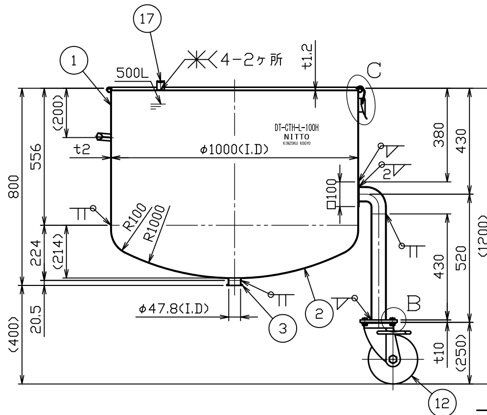
A—A断面图
