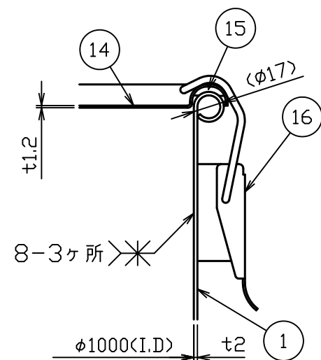
C部詳細図 S = 1 : 3
