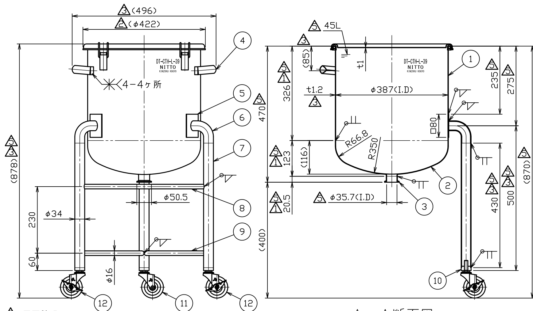
A-A断面図
