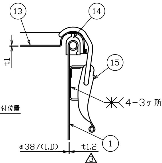
B-B断面図 S=1:2
