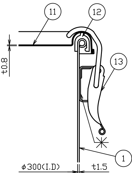
A部詳細図 S=1:2
