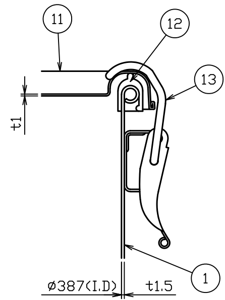
キャッチクリップ詳細図 S = 1 : 2
