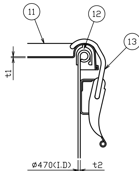
キャッチクリップ詳細図 S = 1 : 2
