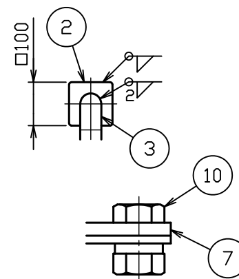
A部詳細図 S = 1 : 2
