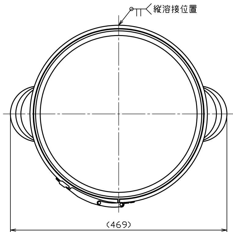
A部詳細図 S = 1 : 1
