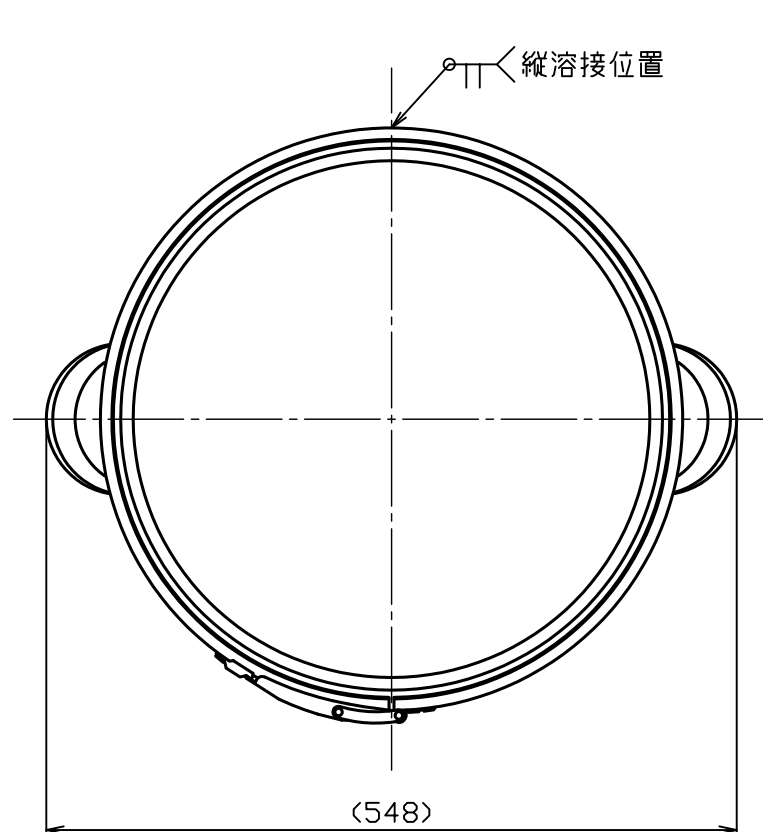
A部詳細図 S = 1 : 1
