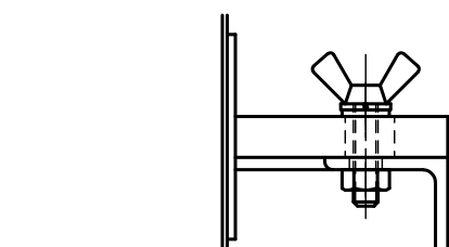
△蝶ボルト部詳細図 S = 1 : 2
