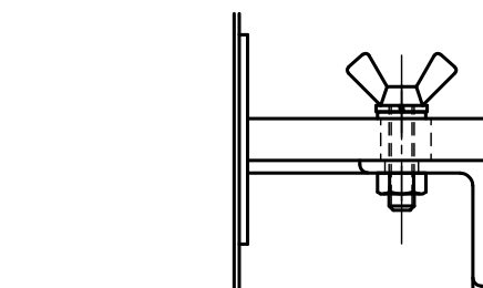
△蝶ボルト部詳細図 S = 1 : 2
