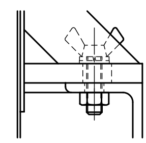
△蝶ボルト部詳細図 S = 1 : 2
