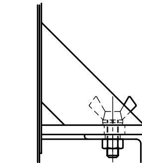
△蝶ボルト部詳細図 S = 1 : 4
