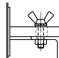
蝶ボルト部詳細図 S = 1 : 2 A部詳細図 S = 1 : 2
