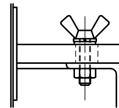
蝶ボルト部詳細図 S = 1 : 2 A部詳細図 S = 1 : 2
