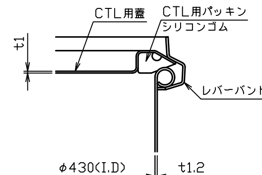
蝶ボルト部詳細図 S = 1 : 2 A部詳細図 S = 1 : 2
