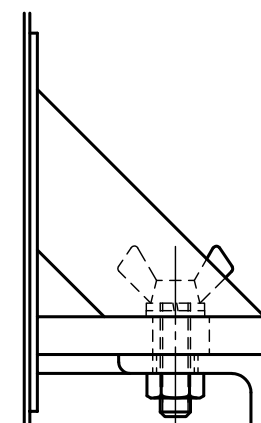
蝶ボルト部詳細図 S = 1 : 2 A部詳細図 S = 1 : 2
