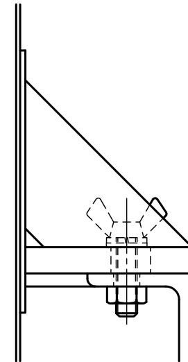
蝶ボルト部詳細図 S = 1 : 2
