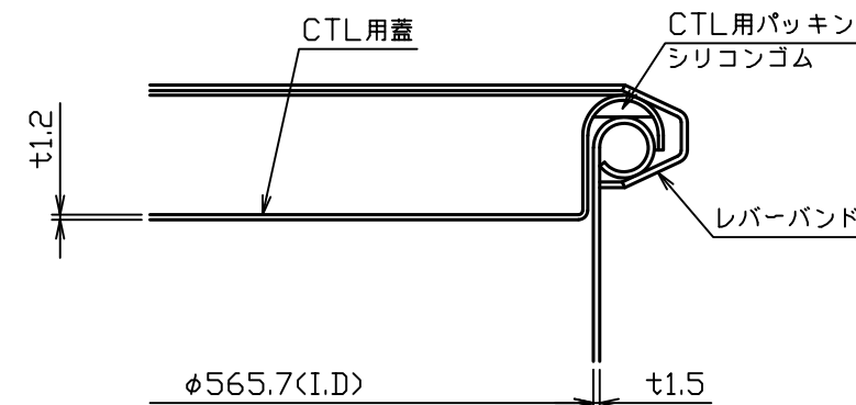
A部詳細図 S = 1 : 2
