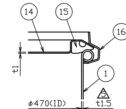
C部詳細図 S=1:2
