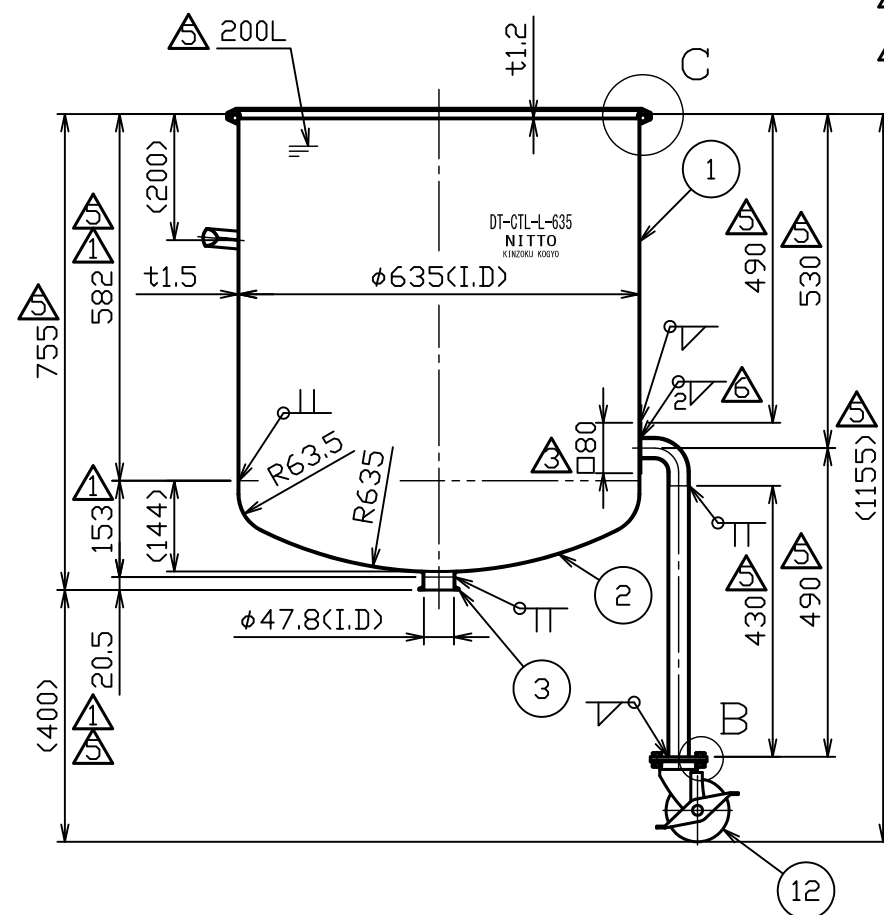
A-A断面図
