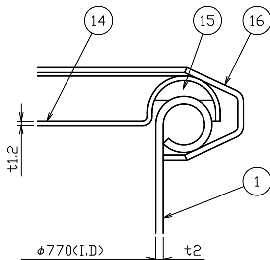
C部詳細図 S = 1 : 1
