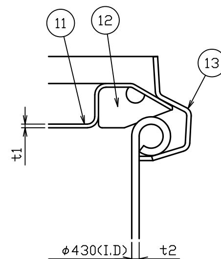
B部詳細図 S = 1 : 1
