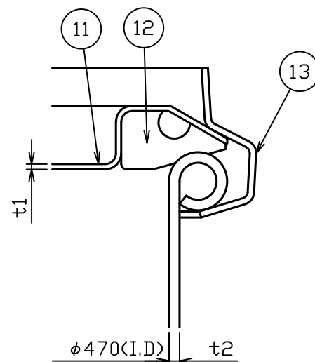
B部詳細図 S = 1 : 1
