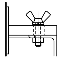
△蝶ボルト部詳細図 S = 1 : 2
