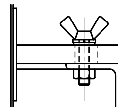
蝶ボルト部詳細図 S = 1 : 2
