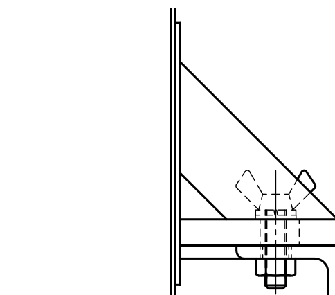
蝶ボルト部詳細図 S = 1 : 2
