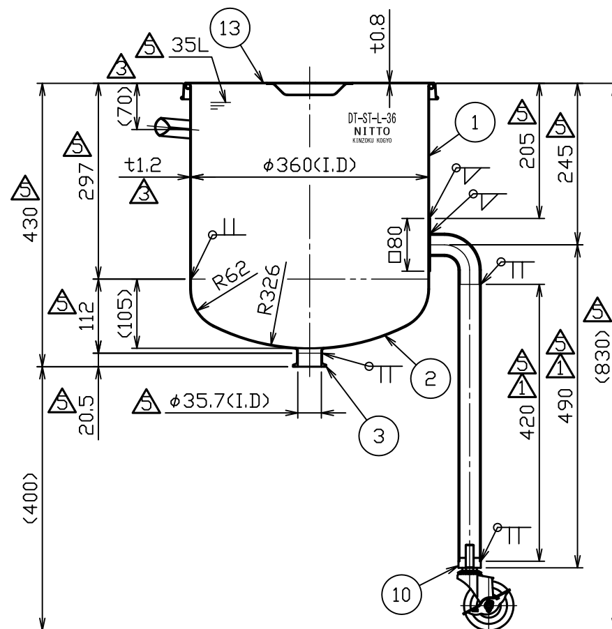
A-A断面図
