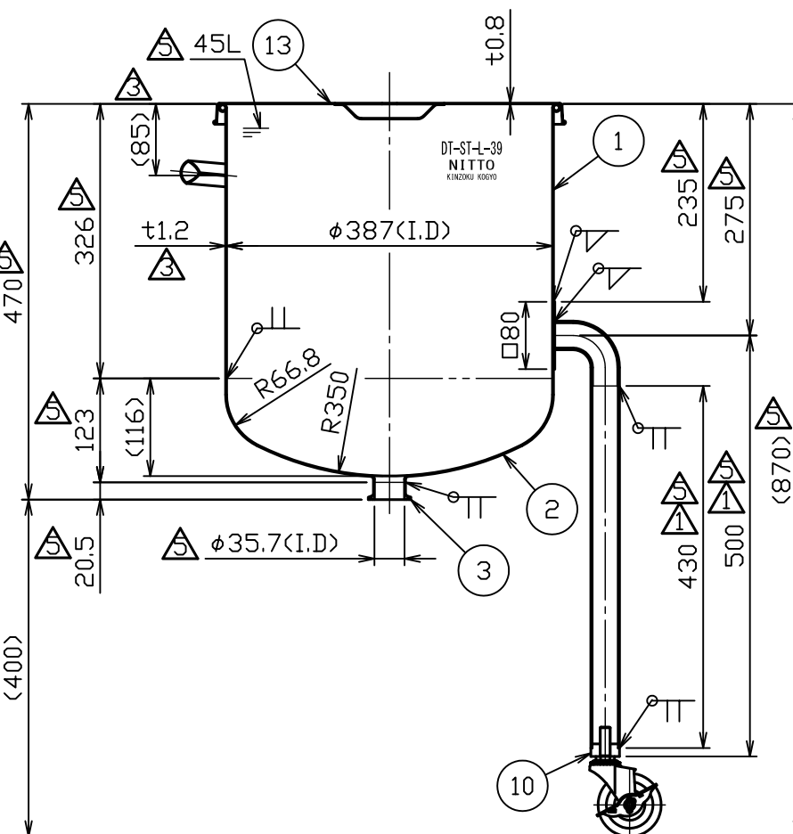
A-A断面図
