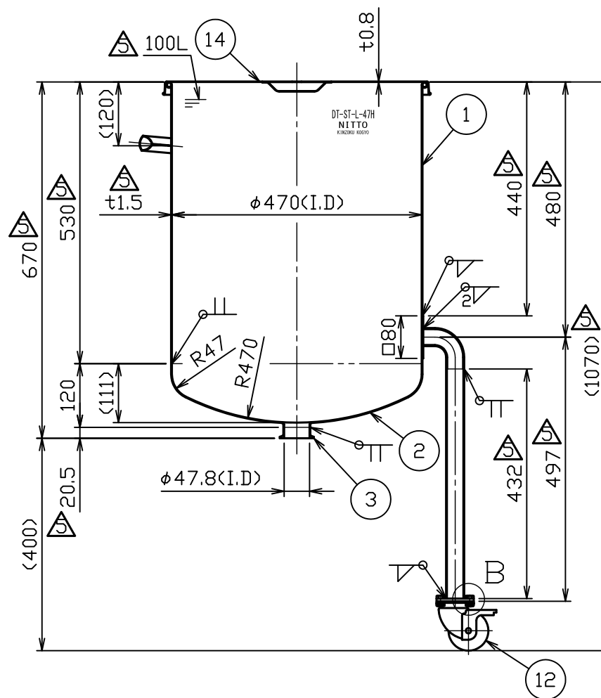
A-A断面図
