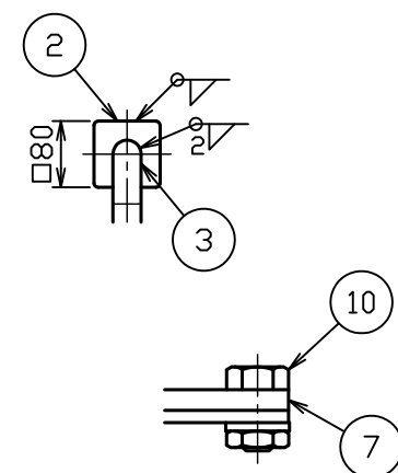
A部詳細図 S=1:2
