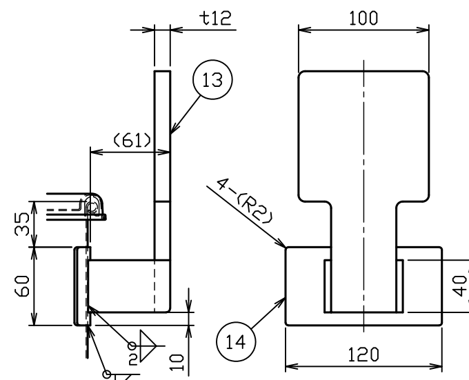
B部詳細図 S = 1 : 4
