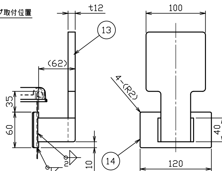
B部詳細図 S = 1 : 4
