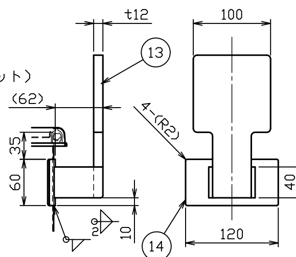
A部詳細図 S = 1 : 5
