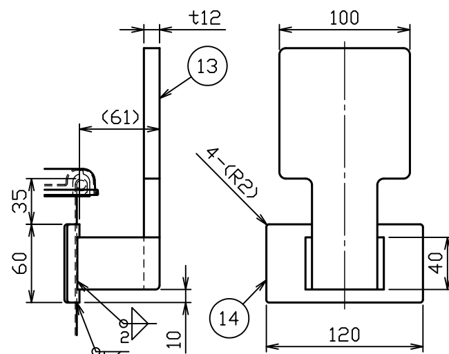
A部詳細図 S = 1 : 4
