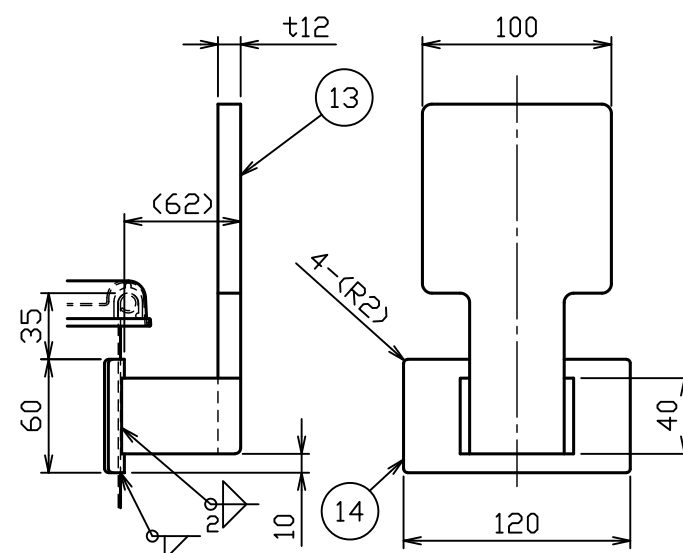
A部詳細図 S = 1 : 4
