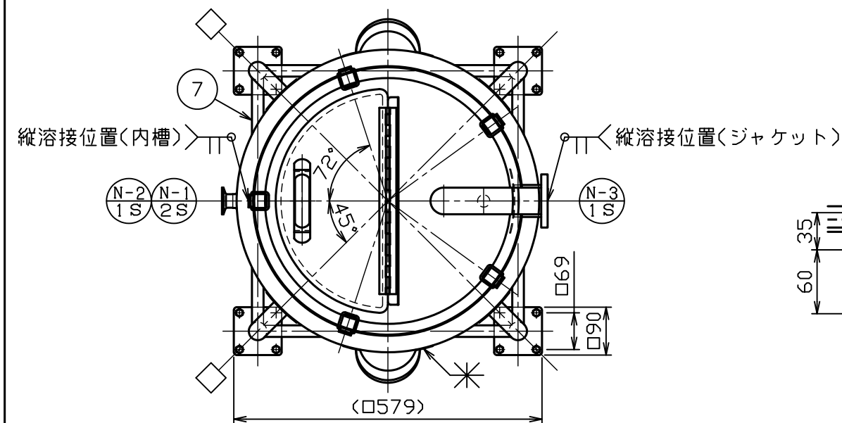
A部詳細図 S = 1 : 5
