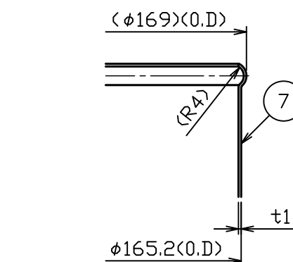
短管部詳細図 S = 1 : 2
