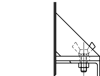
△蝶ボルト部詳細図 S = 1 : 4
