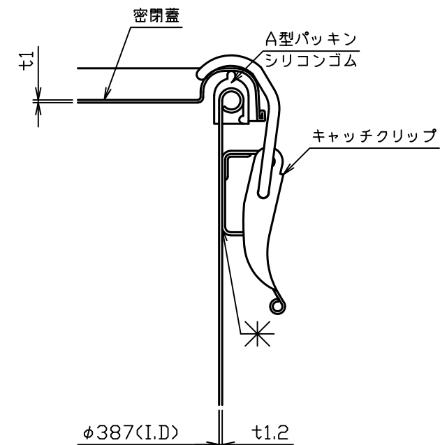
A部詳細図 S = 1 : 2
